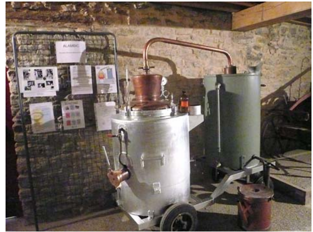
Alambic avec ses accessoires. A été réformé le 07/12/2022
